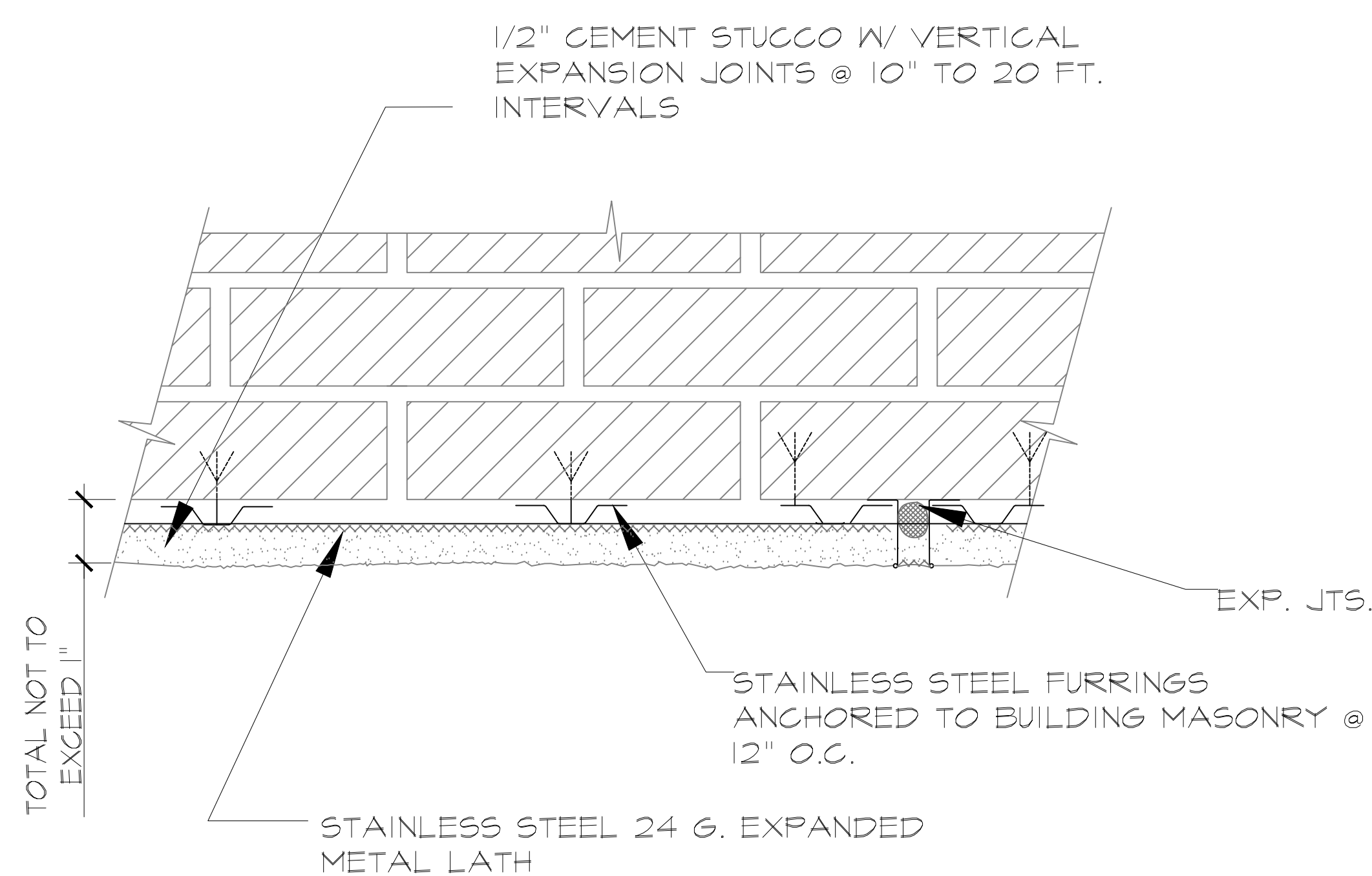
3 STUCCO DETAILS A-206 SCALE: 1/8" = 1'-0"
