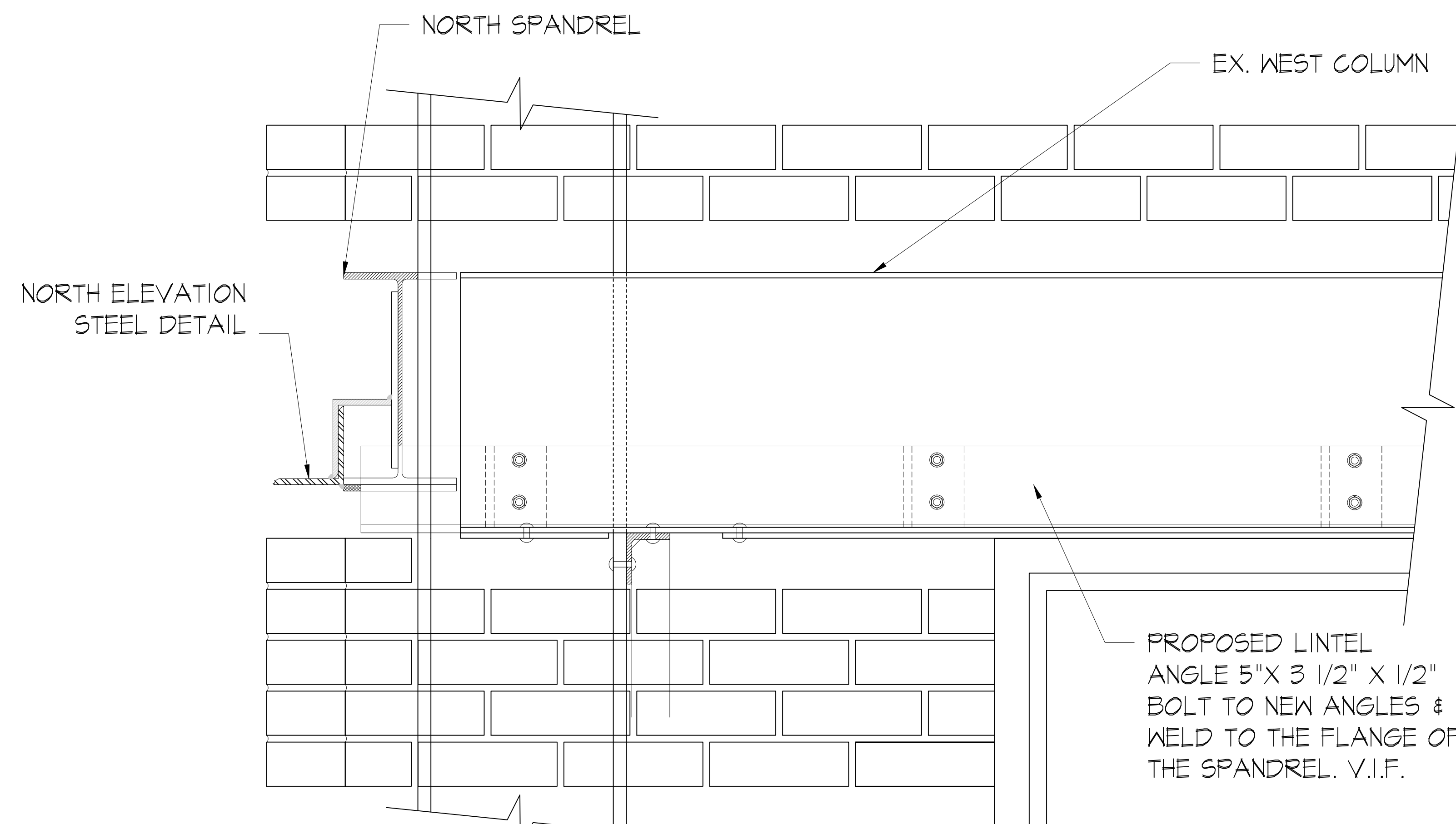
5 PROPOSED REPAIR DETAIL - ELEVATION A-205 SCALE: N.T.S.
