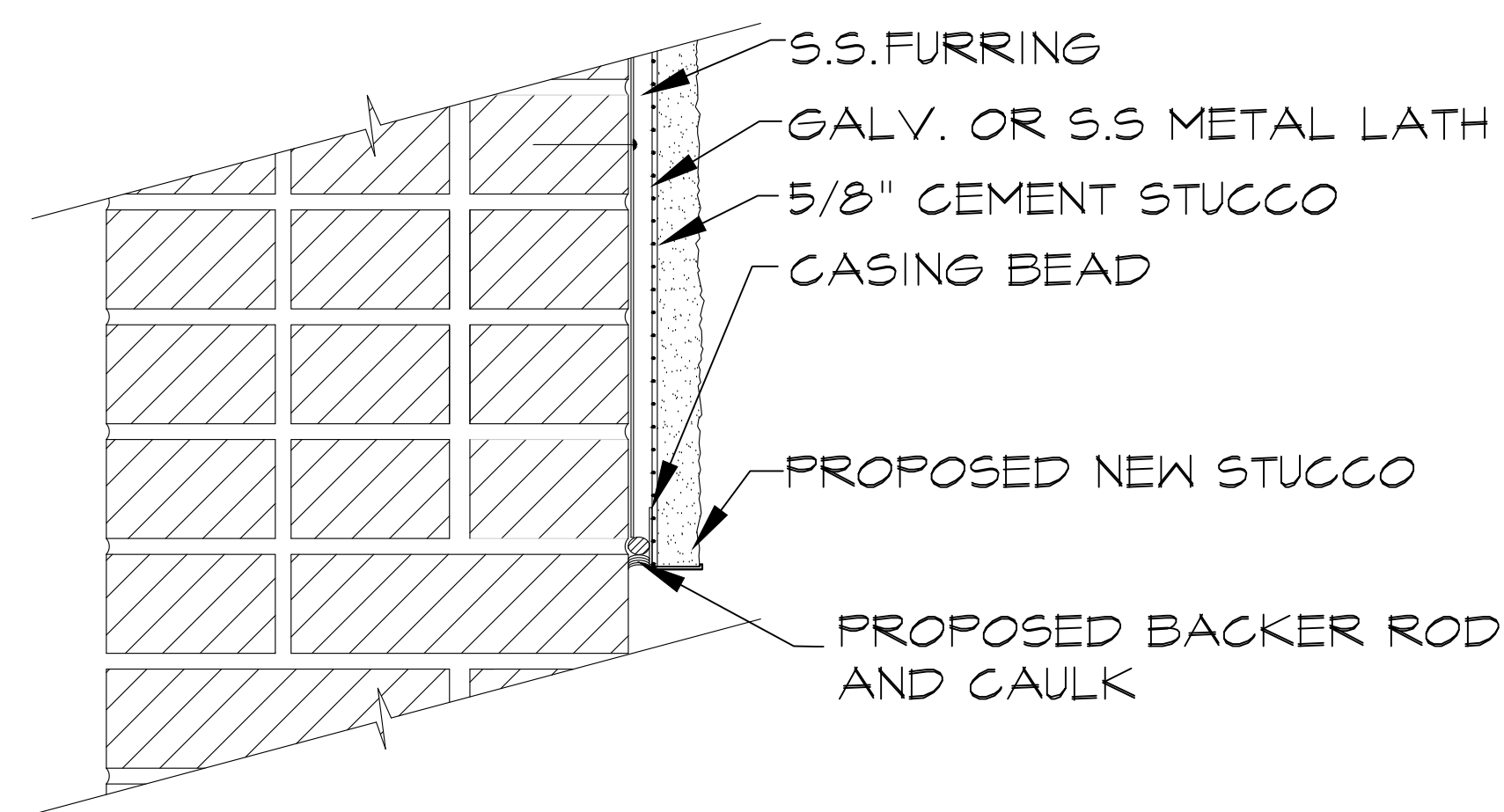
4 STUCCO DETAILS - BOTTOM TERMINATION A-204 SCALE: 3"=1'-0"
